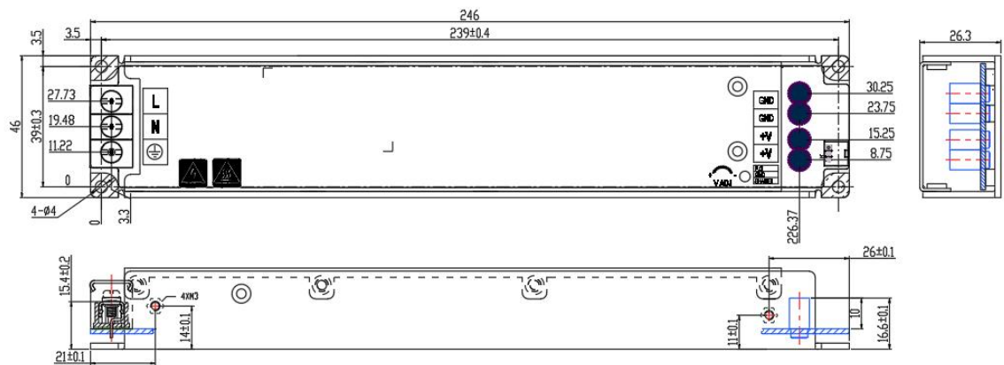
输入、输出端子定义及安装注意事项
